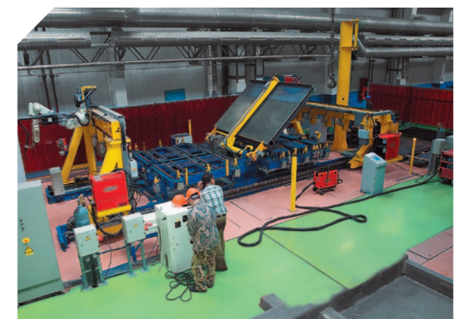
Встроенный кантователь книжного типа
