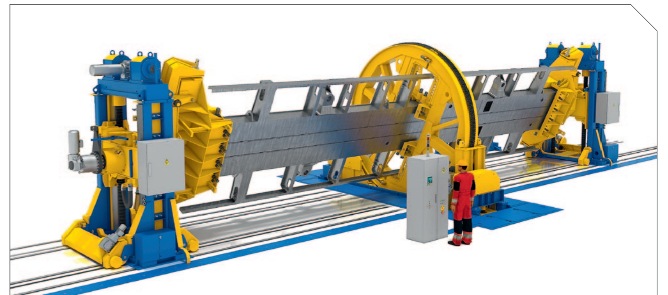
Кантователь с подъемными центрами грузоподъемностью 40 т
